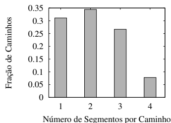
Fig. 4. Distribuição da quantidade de segmentos por caminhos calculados em f_3(x) .
